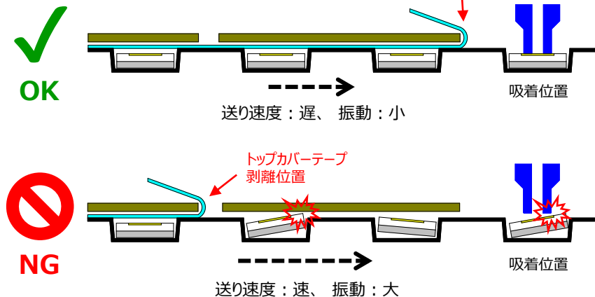
図4. トップカバーテープ剥離位置について
