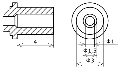
図2. 推奨吸着ノズル形状
