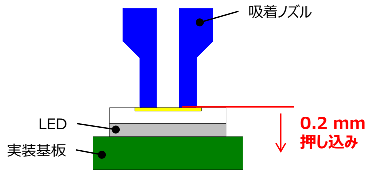
図6. 推奨搭載高さ
