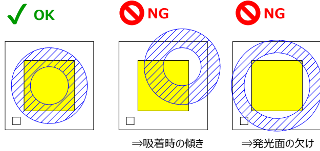
図3. 吸着位置について
